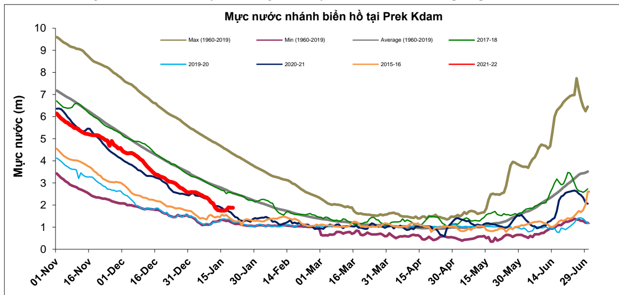
Hình 1. Diễn biến nước trạm Prek Kdam - Biển hồ, cập nhật ngày 20/01/2022
