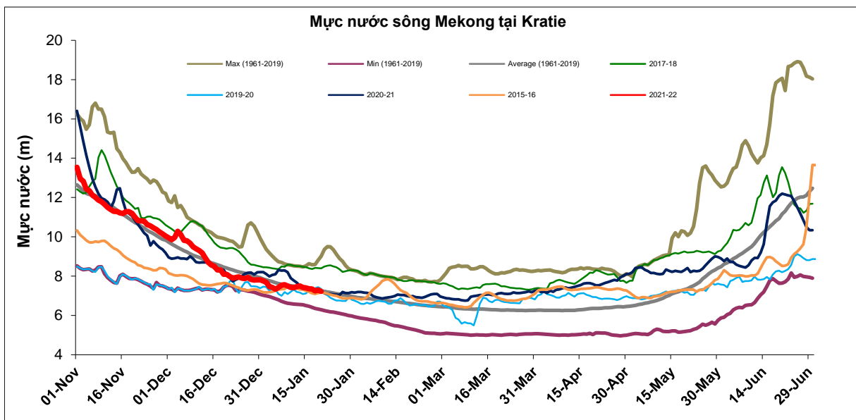
Hình 3. Diễn biến mực nước về qua trạm Kratie, cập nhật ngày 20/01/2022
