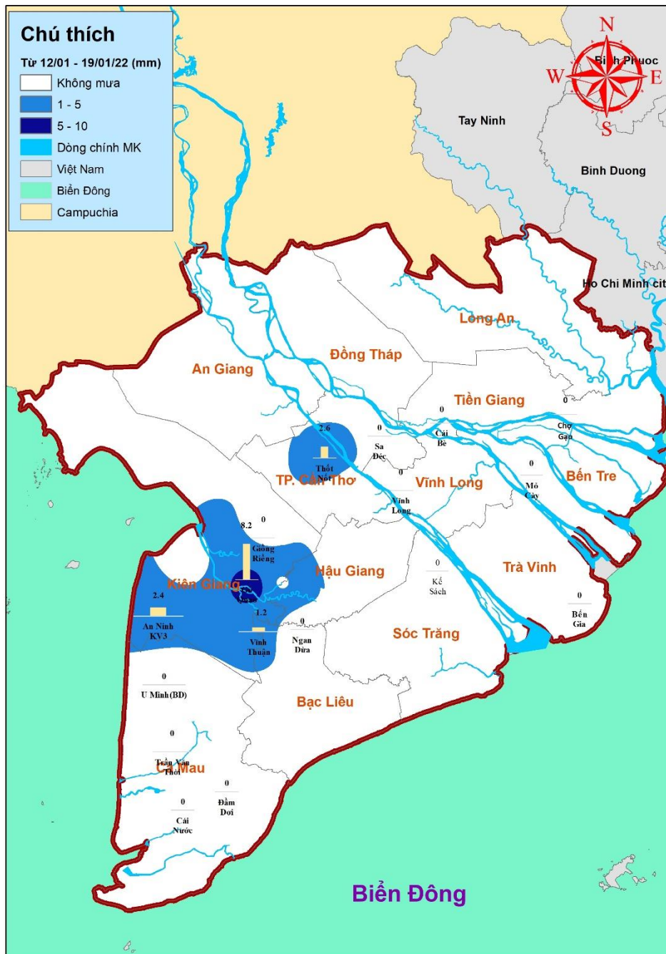
Hình 4. Bản đồ lũy tích lượng mưa trên ĐBSCL (từ ngày 12/01 đến 19/01/2022)
