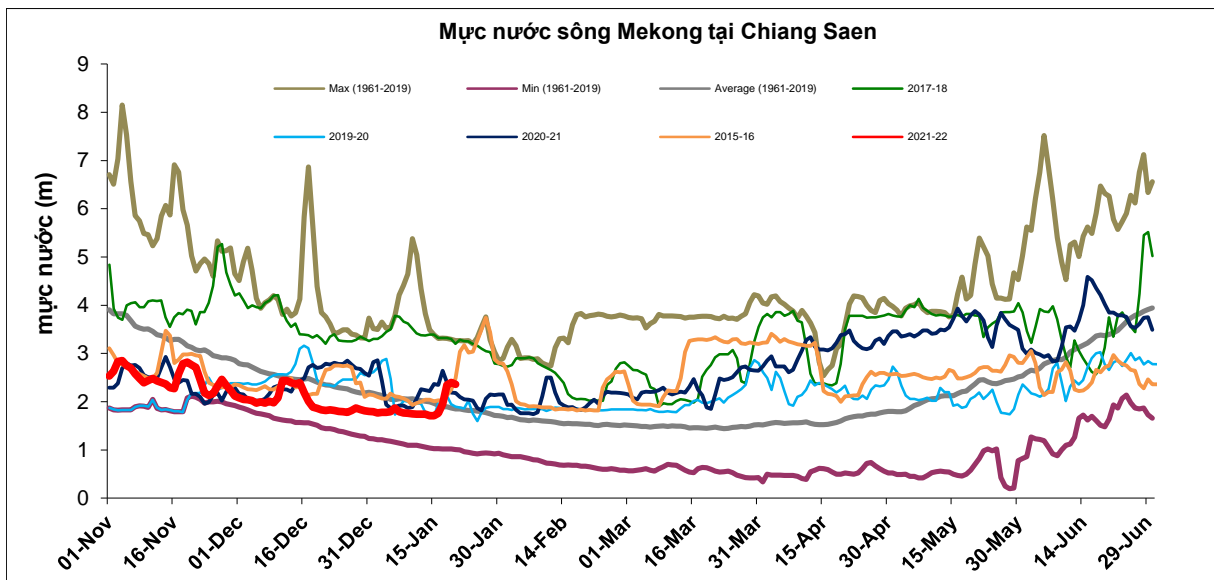
Hình 2. Diễn biến mực nước tại Chiang Saen –Thái Lan, cập nhật 20/01/2022
